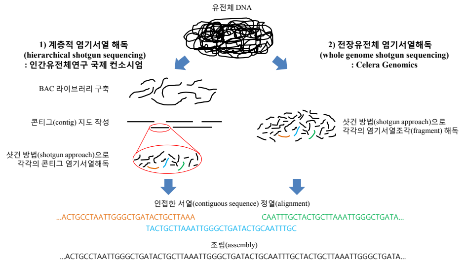
<그림 6> HGP에서 사용된 염기서열 해독 전략
