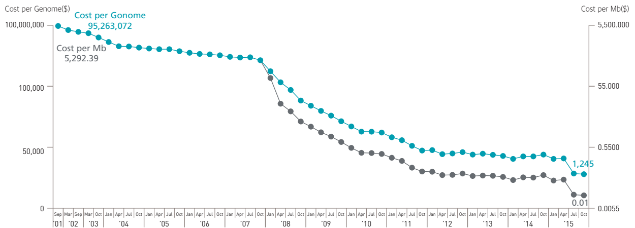
<그림 2> 유전체 해독 비용
